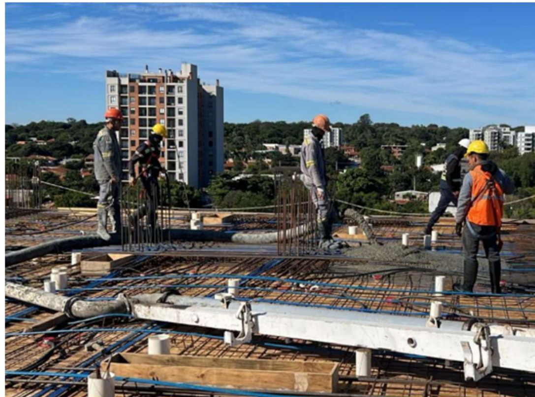
Cargamento de Pilares N10-N11 – Cargamento de Losa N10
